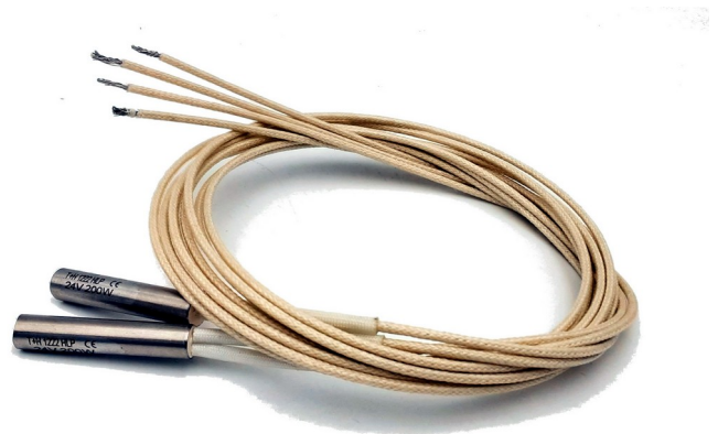
Abbildung 1 links: NEO9XXHT-Sensor mit 8mm Bohrungen für Heizkartuschen Abbildung 1 rechts: NEO20X-Heizkartuschen
