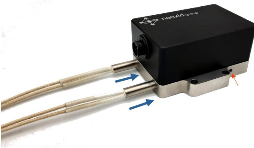
Abbildung 2: NEO9XXHT-Sensor mit halbreingesteckten Heizkartuschen NEO203
