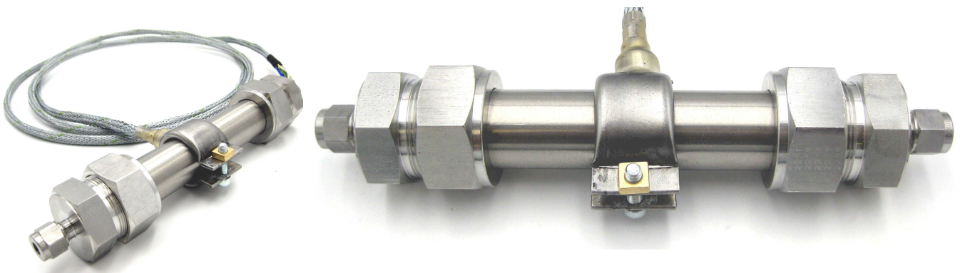
Abbildung 1: H 2 -Brenner Version NEO305 mit Heizband und optionalen Adapter auf 6mm Klemmringverschraubung
