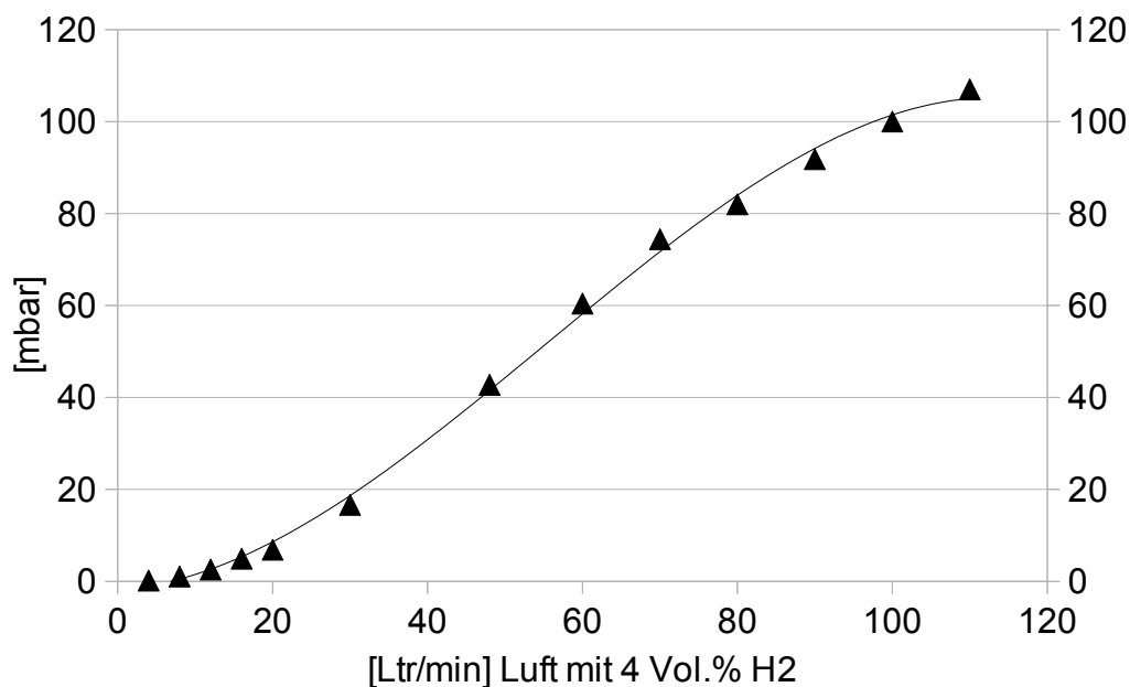
Abbildung 2: Gegendruck bei Umsatz von 4 Vol.% H 2 in Luft, 20°C Eingangstemperatur
