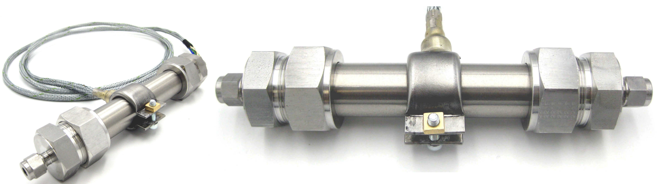
Abbildung 1: H 2 -Brenner Version NEO305 mit Heizband + optionalen Adapter auf 6,35mm Klemmringverschraubung
