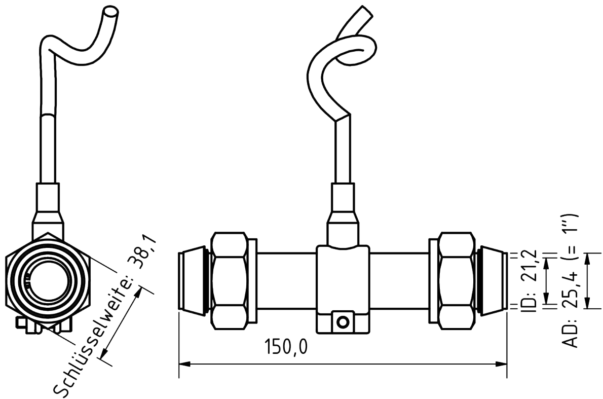
Abbildung 2: Anschlussmaße vom Gehäuse mit Heizung und 1" Klemmringverschraubung
