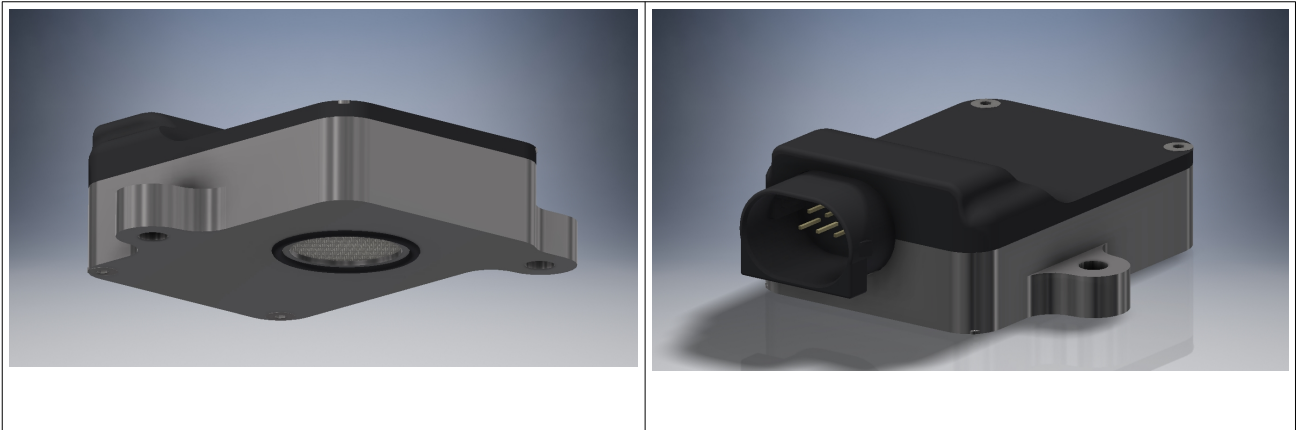
Abbildung 1b: H 2 -Sensorsystem NEO10XX Serie von unten
