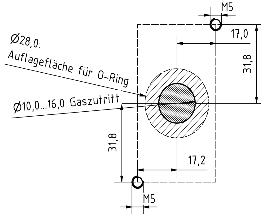
Abbildung 3b: Bohrschablone
