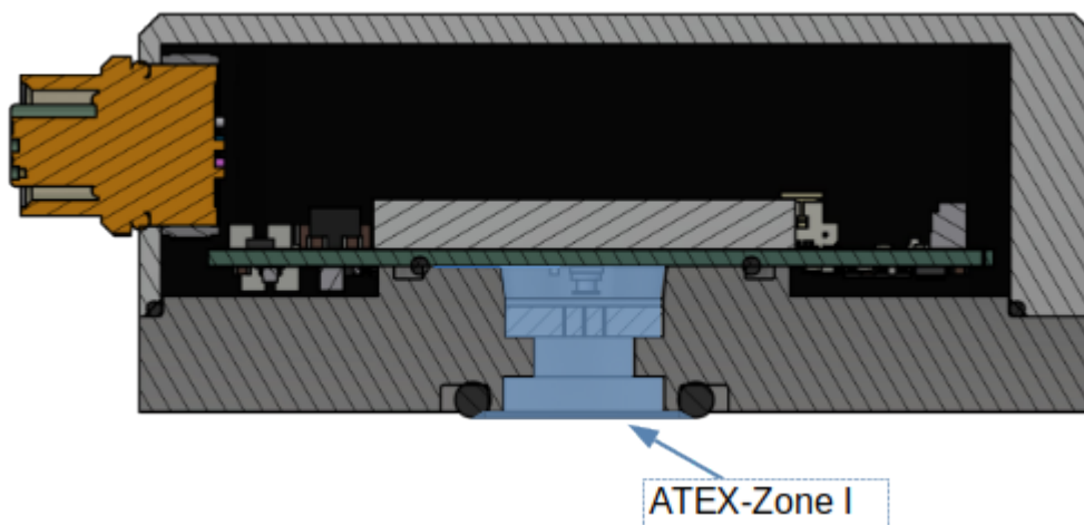
Abbildung 2a: Bereich ATEX Zone I
