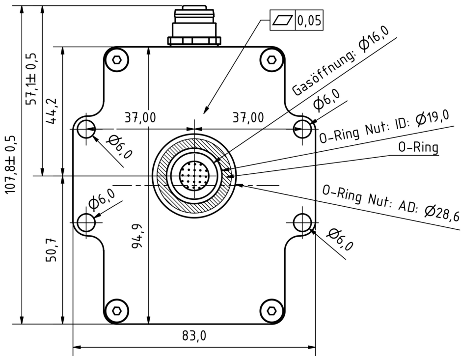
Abbildung 3a: Lochbild vom H 2 -Sensorsystem von unten
