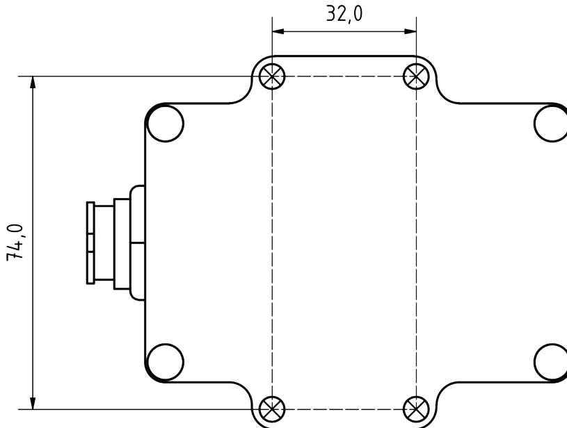
Abbildung 3b: Bohrschablone
