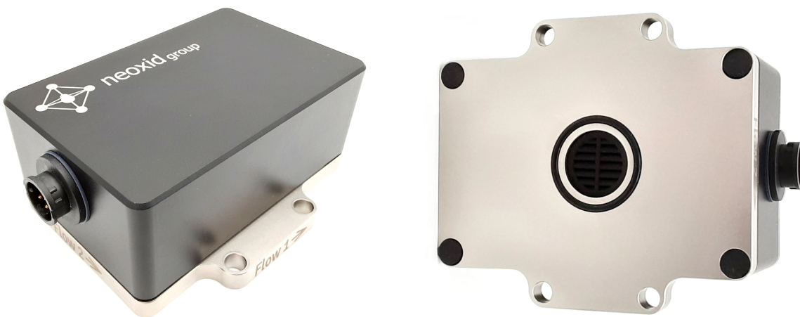
Abbildung 1: H 2 -Konzentrationssensor Version NEO962
