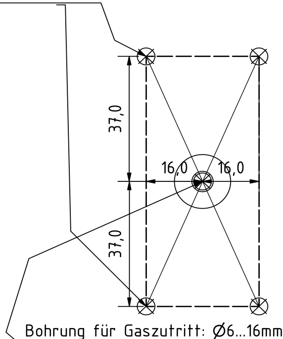
Abbildung 3b: Bohrschablone
