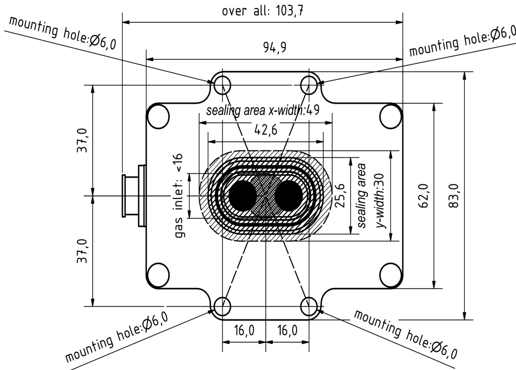
Abbildung 3a: Lochbild vom H 2 -Sensorsystem von unten
