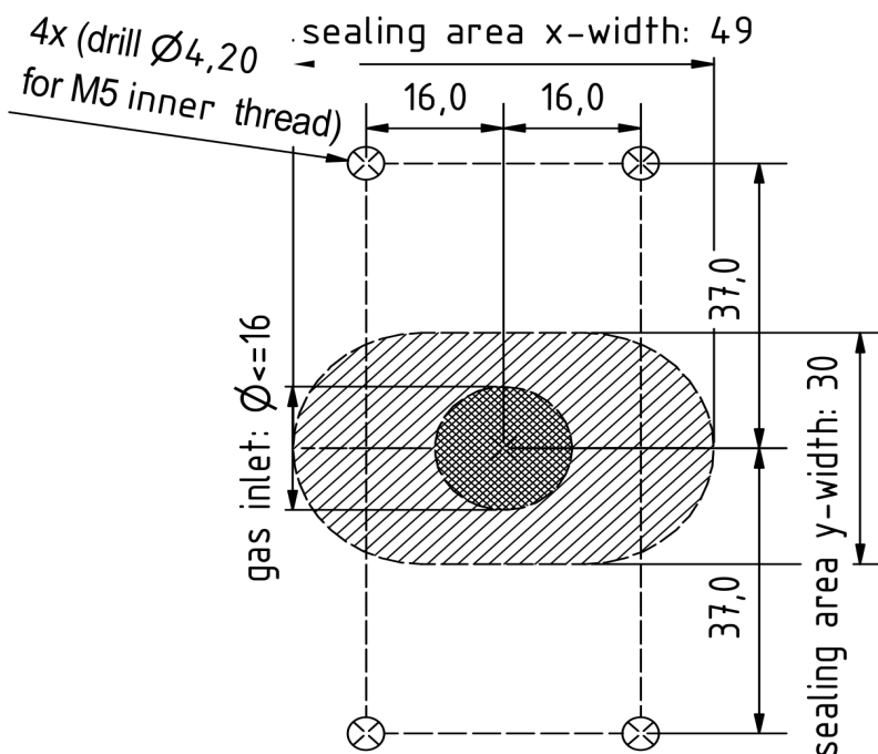
Abbildung 3b: Bohrschablone
