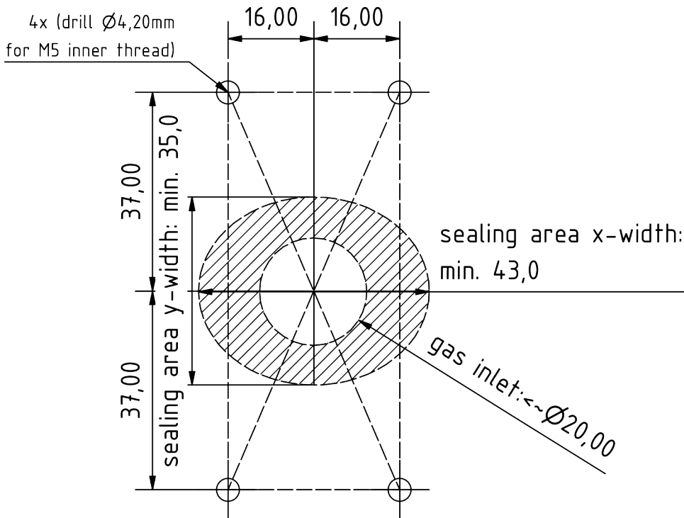
Abbildung 3b: Bohrschablone
