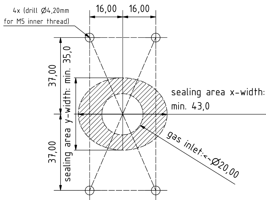
Abbildung 3b: Bohrschablone
